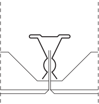
Dalle Sicilia Clip-In Biseau 3 mm
