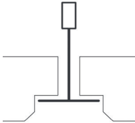
Ossature visible Décaissé K5-FS
