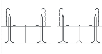
Ossature cachée Vissé K0
