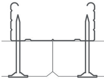
Profilé caché Vissé K5
